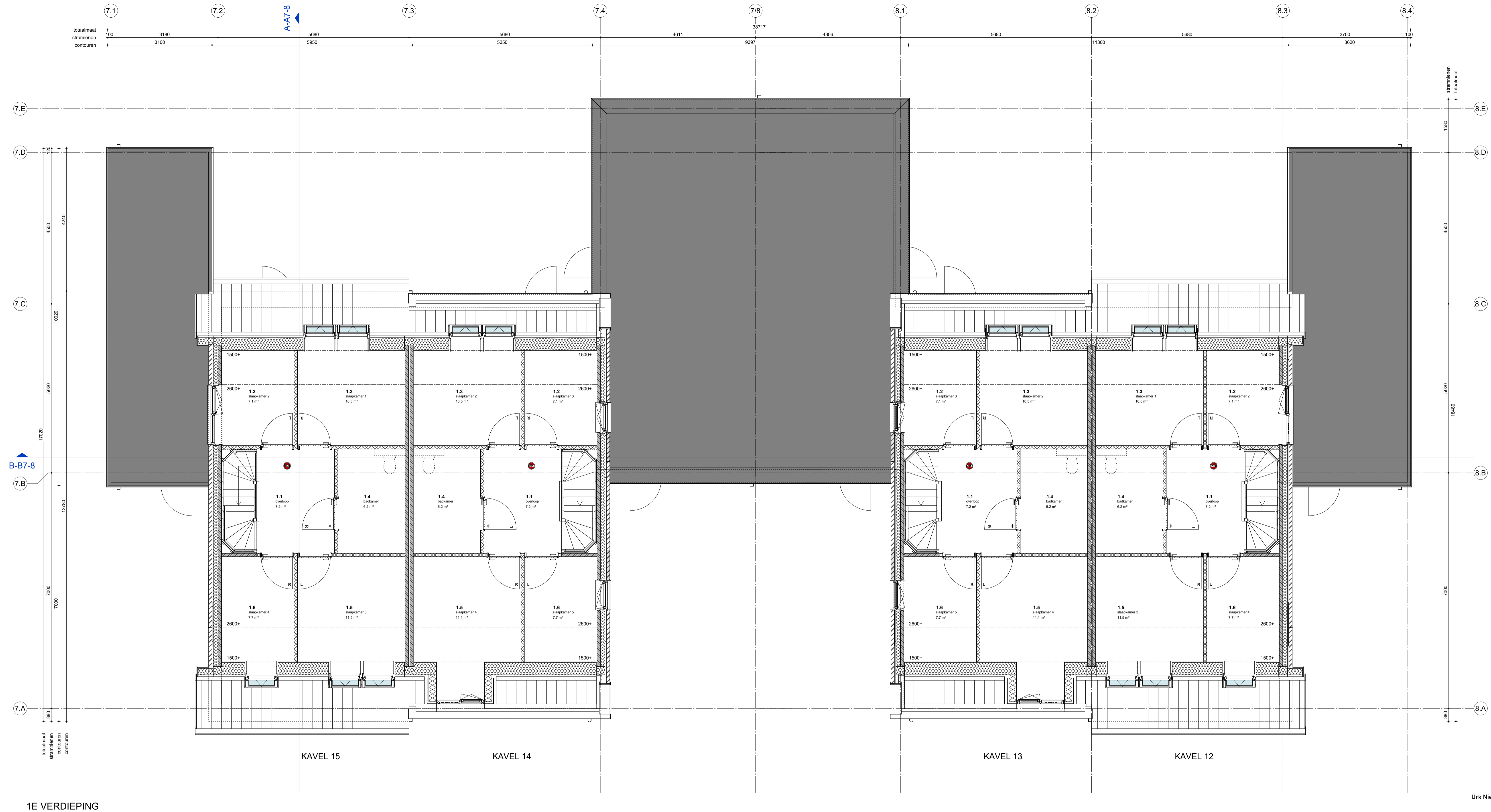
1E VERDIEPING
