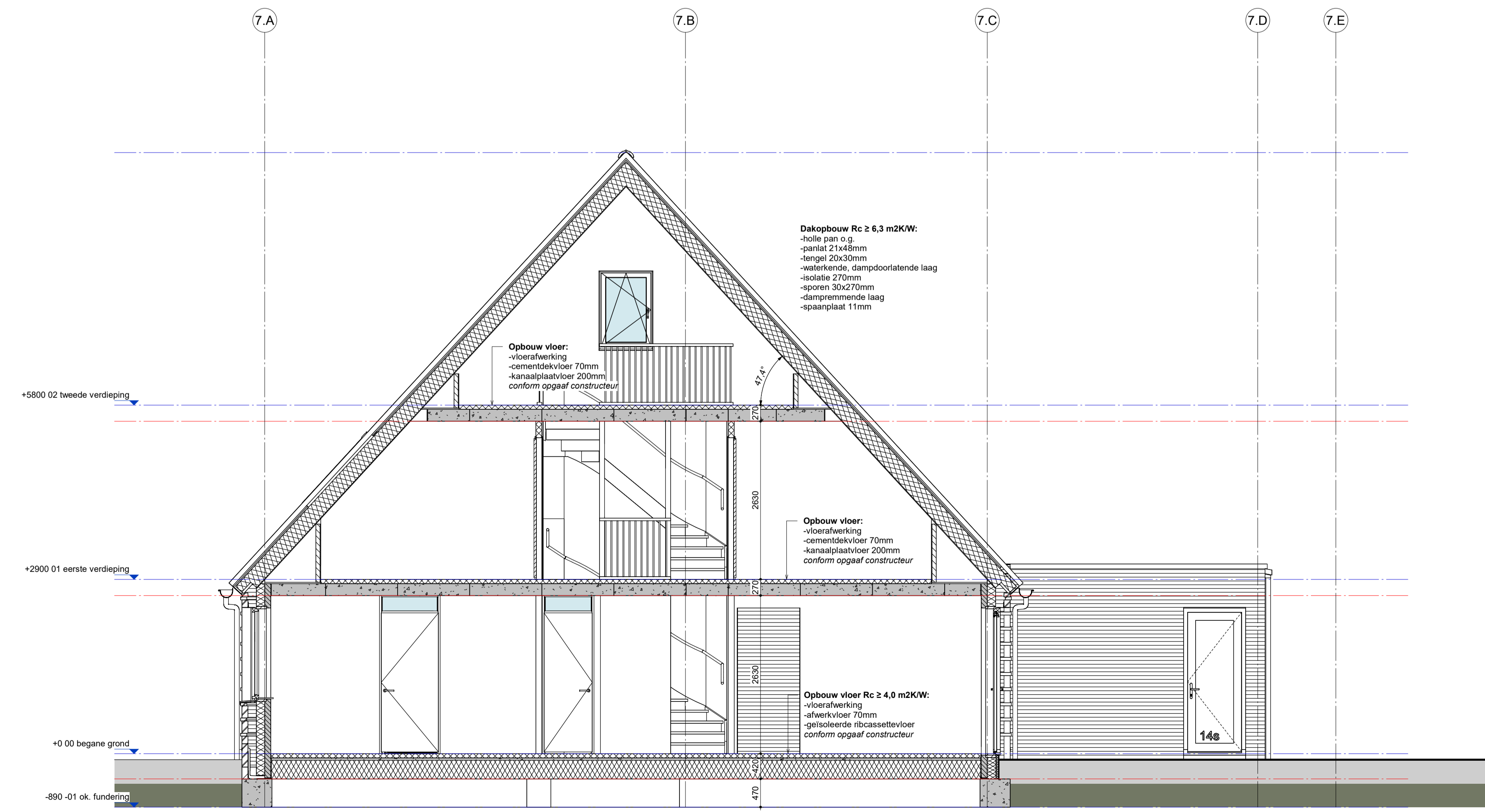
DOORSNEDE A
